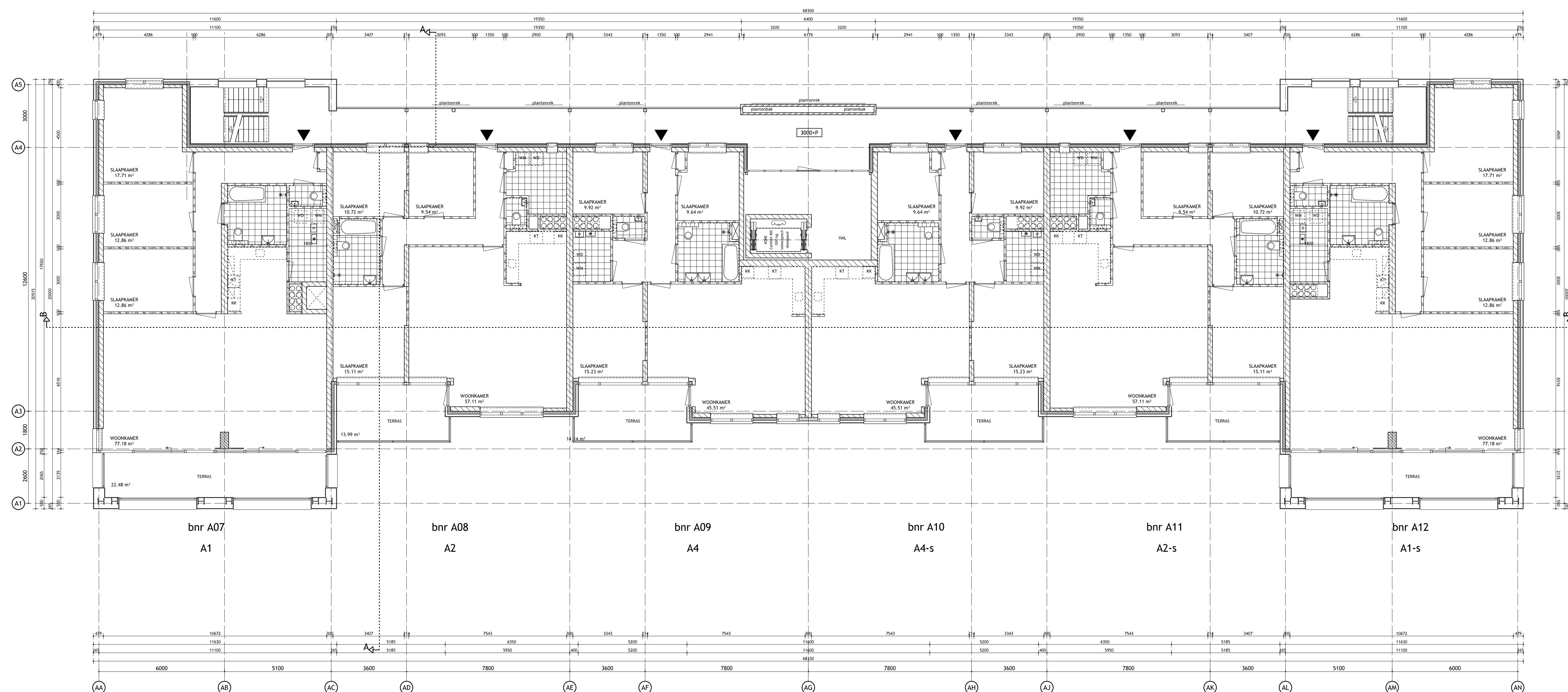
1e verdieping gebouw A
