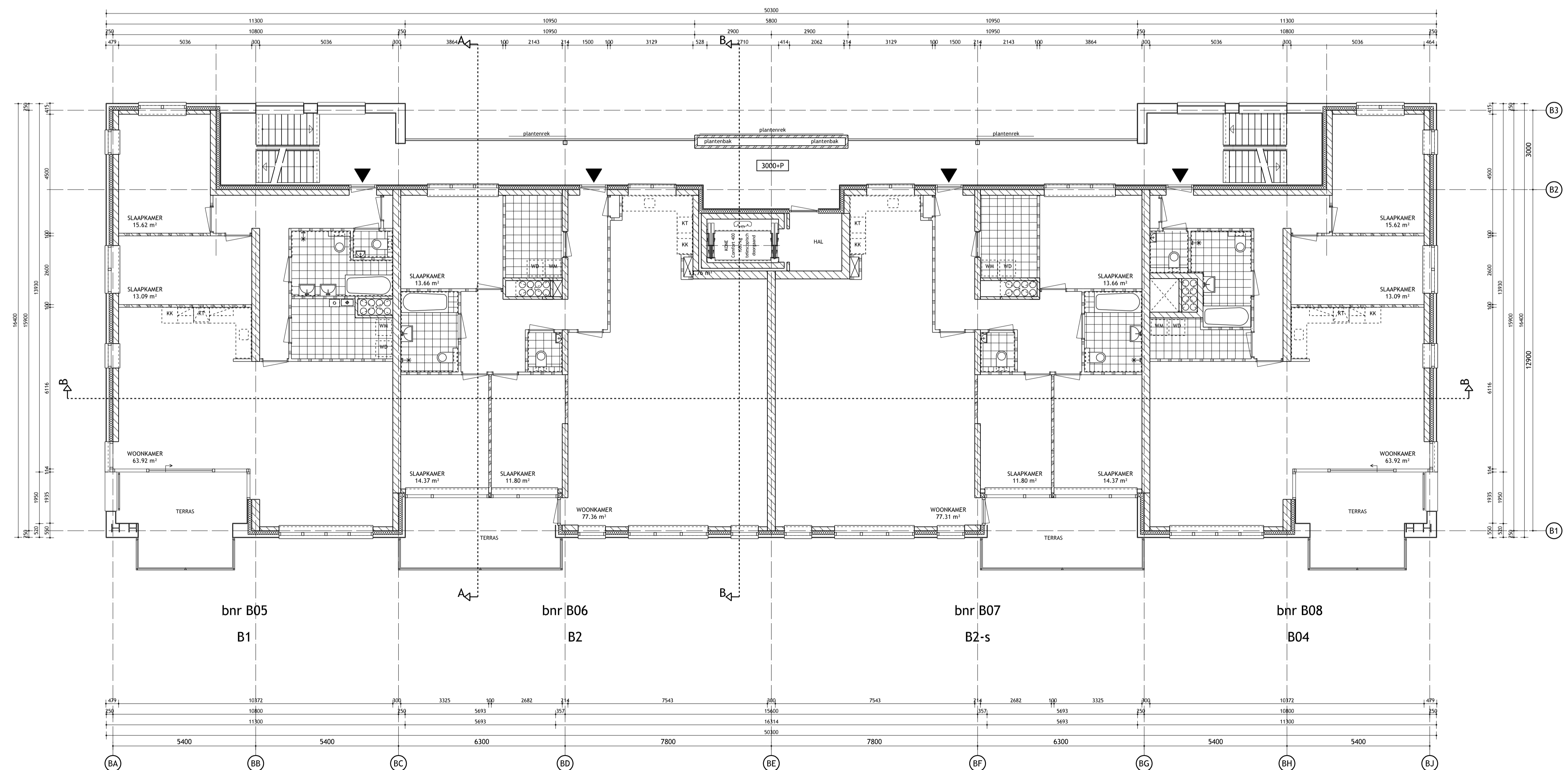
1e verdieping gebouw B
