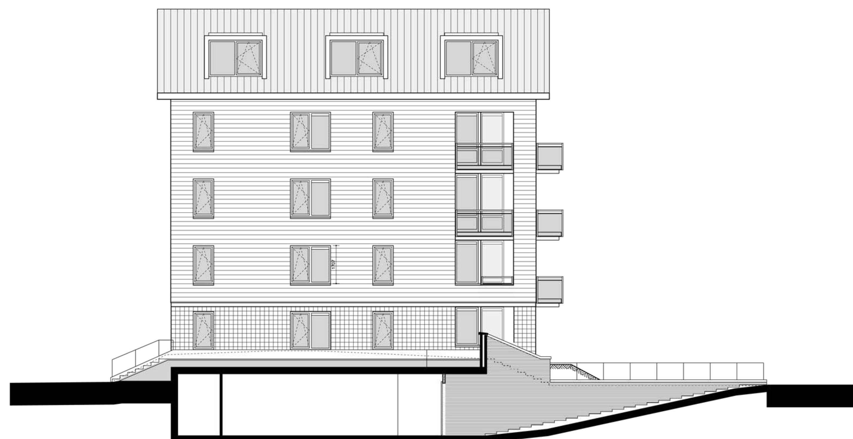
Linkerzijgevel / gebouw B
