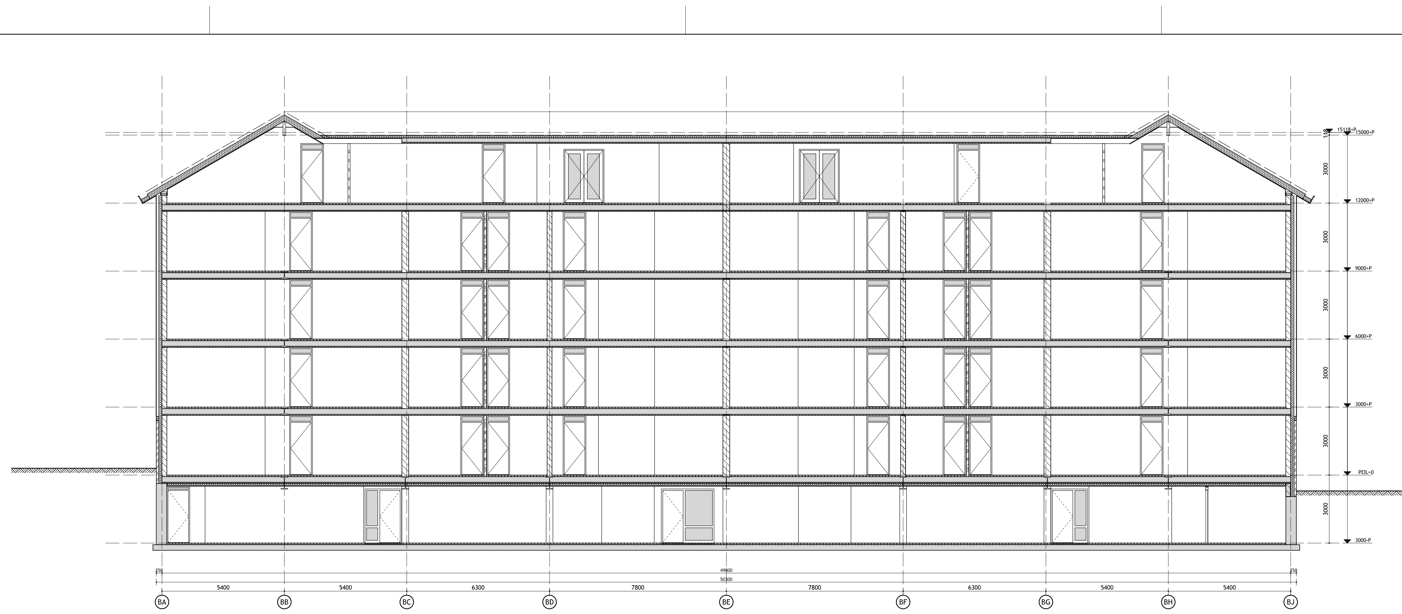
DOORSNEDE B-B
