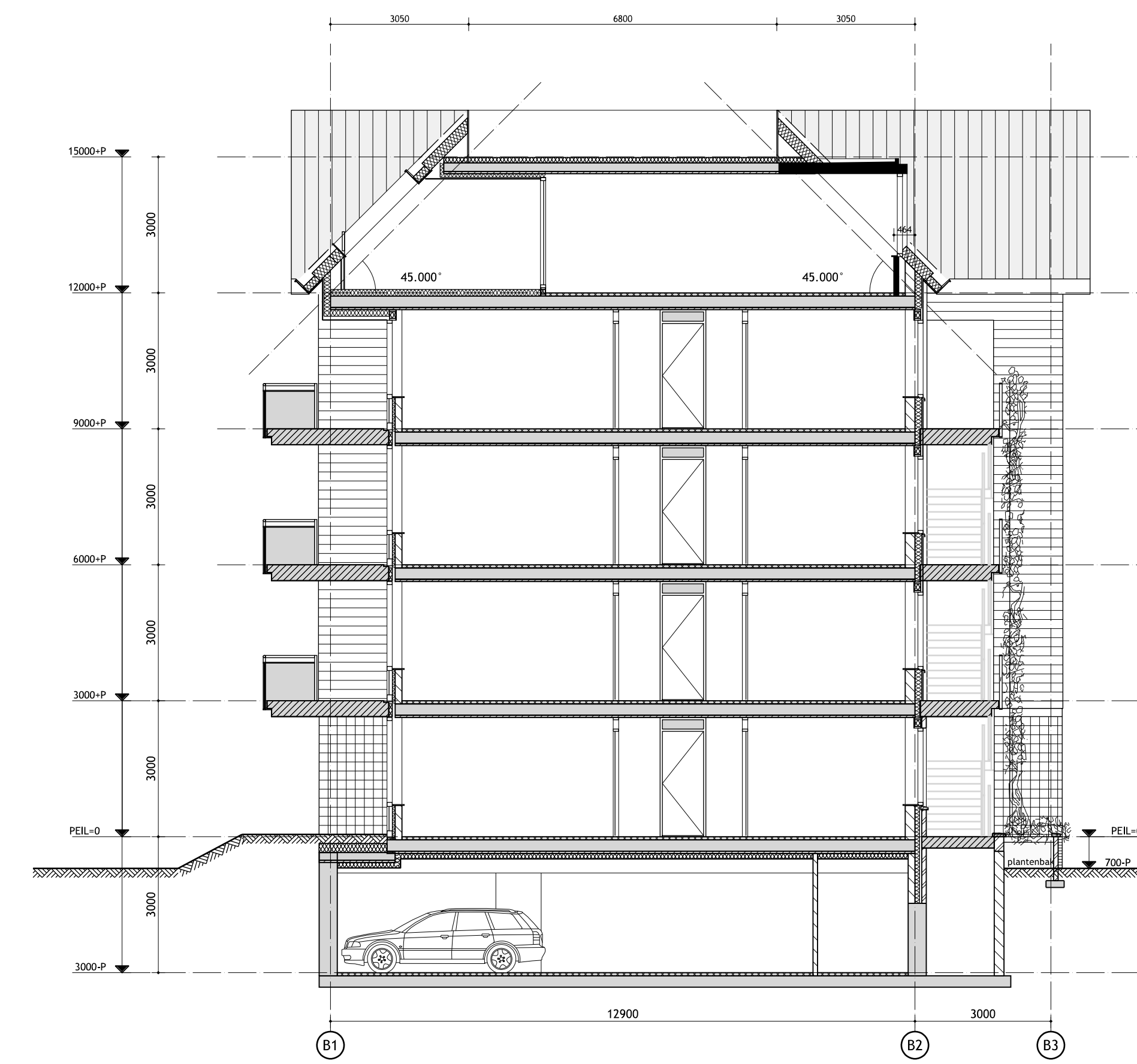
DOORSNEDE A-A
