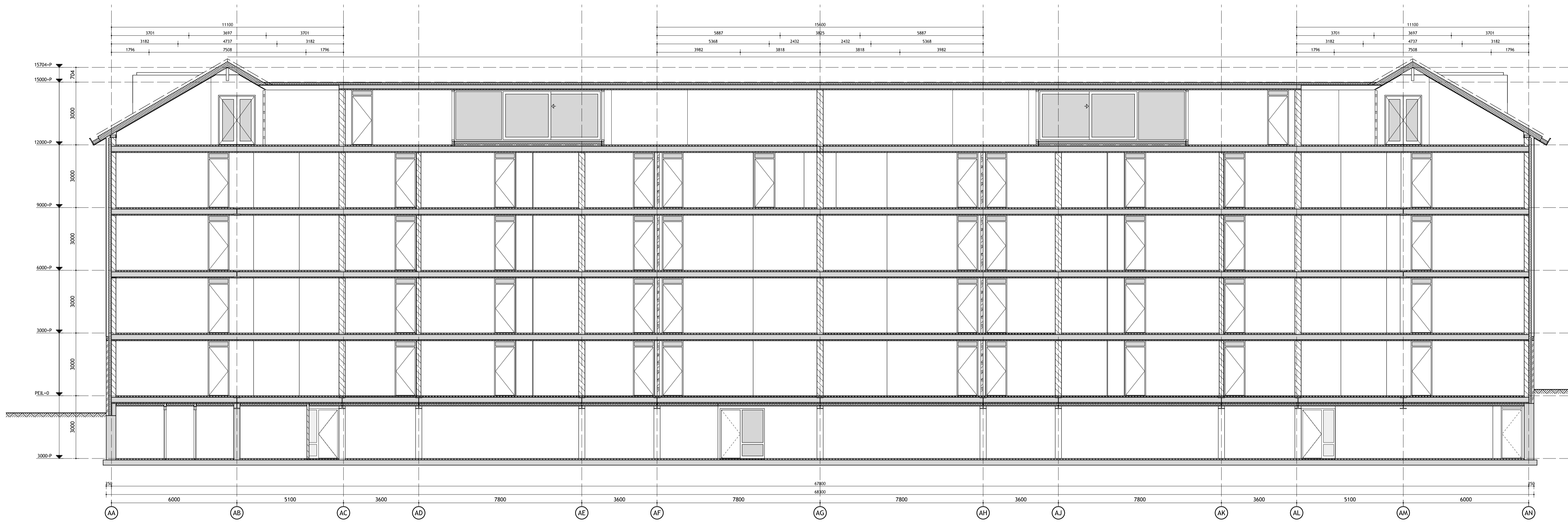
DOORSNEDE B-B
