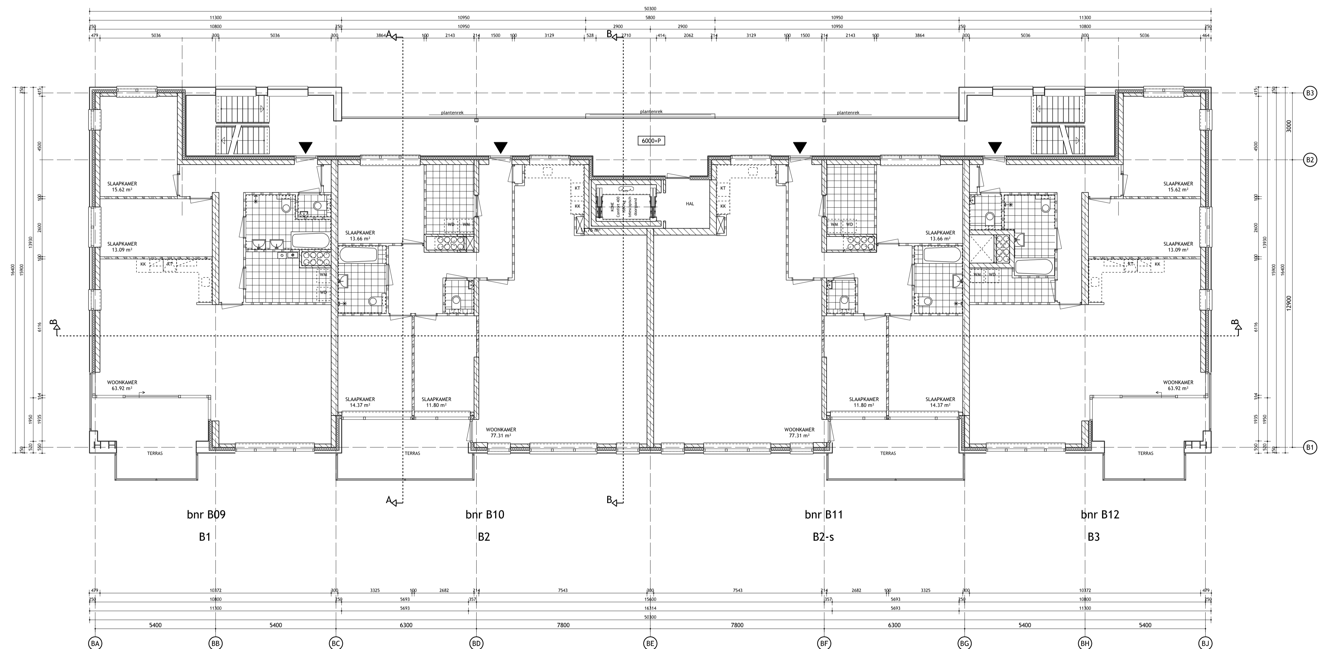
2e Verdieping gebouw B
