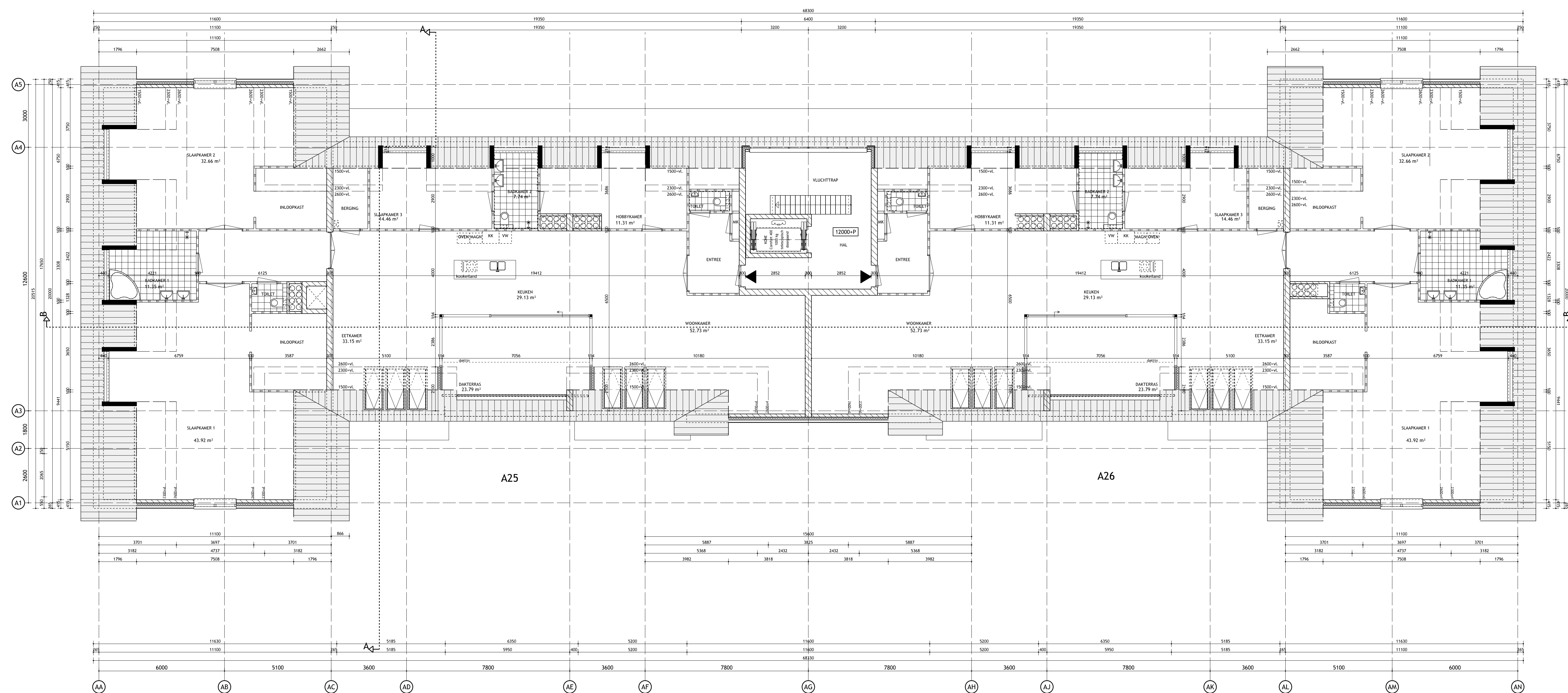
4e verdieping gebouw A
