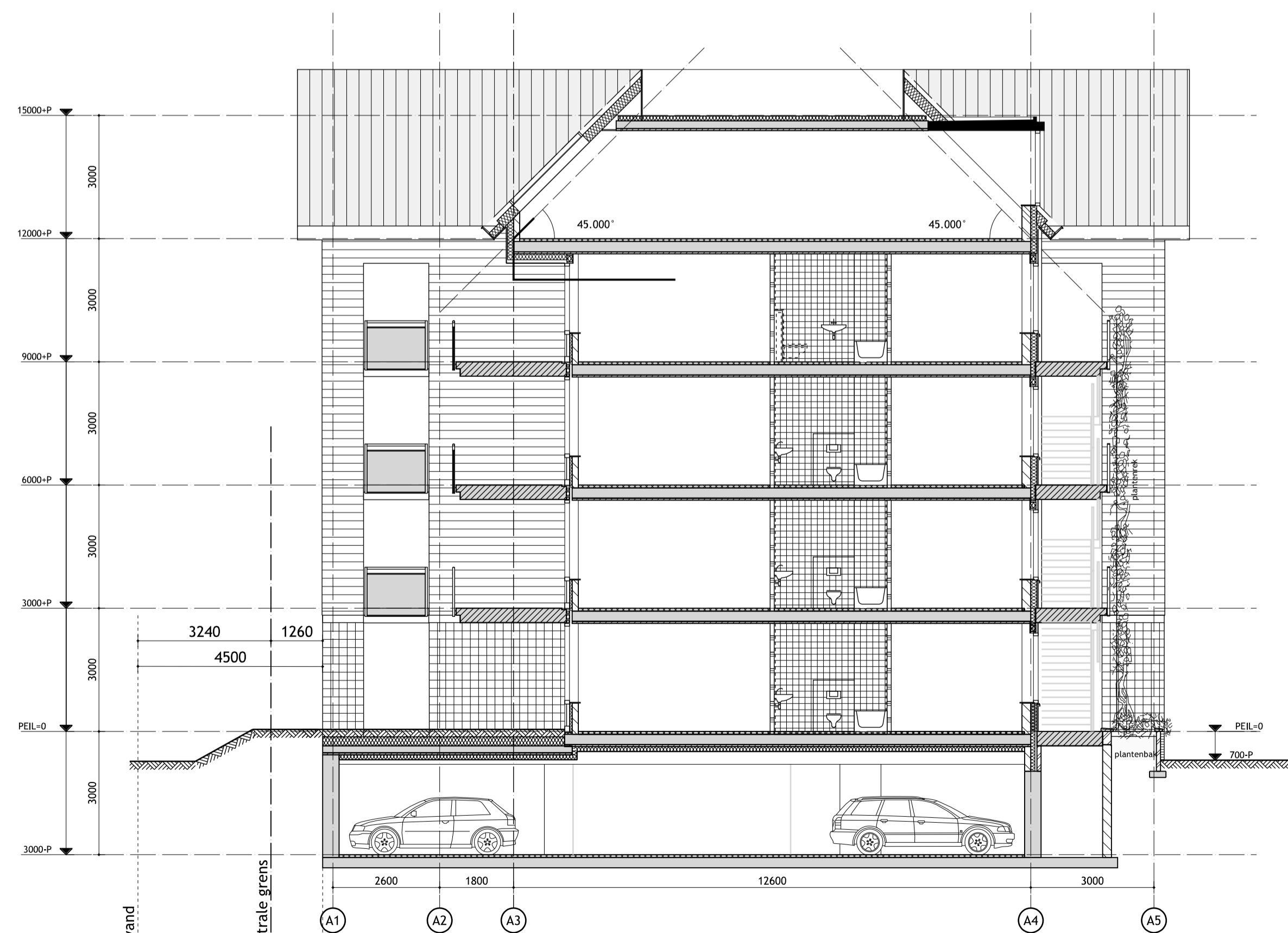
DOORSNEDE A-A
