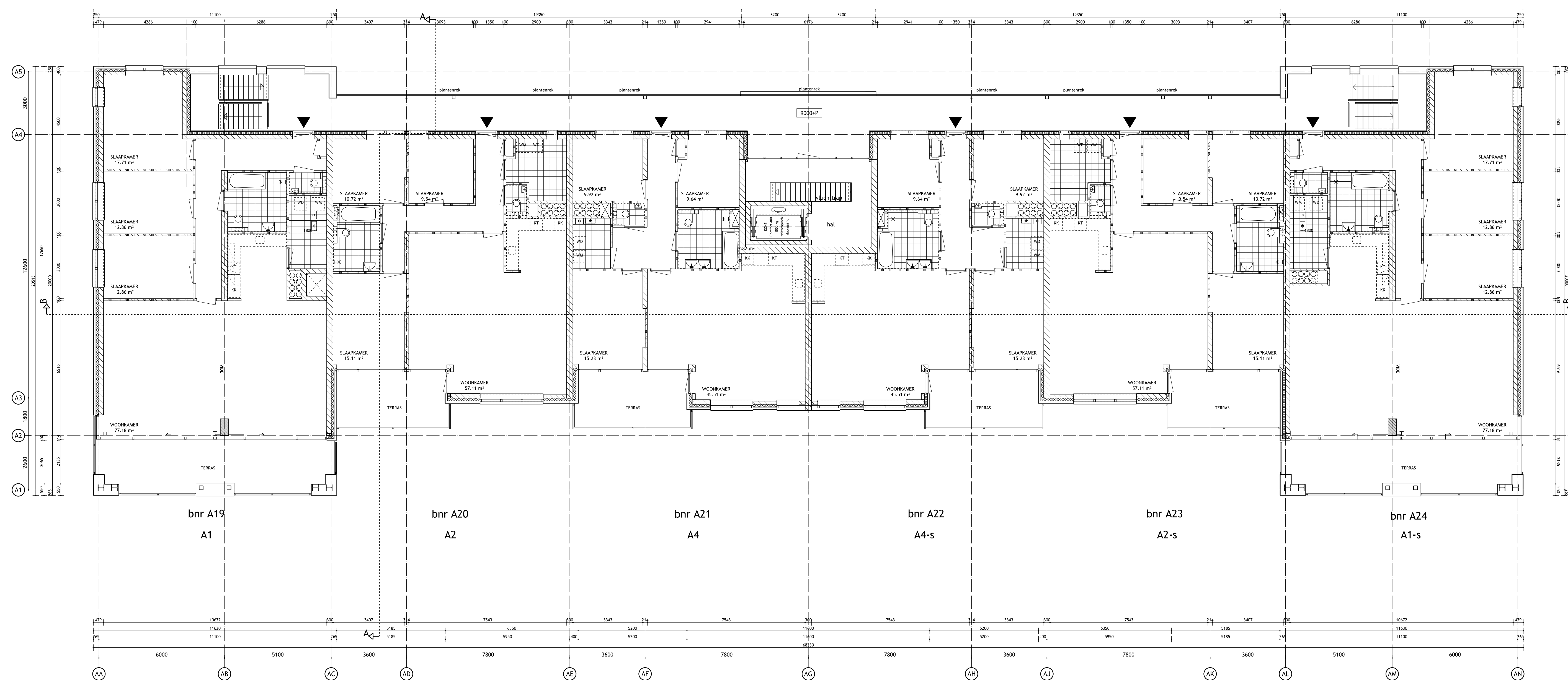
3e verdieping gebouw A
