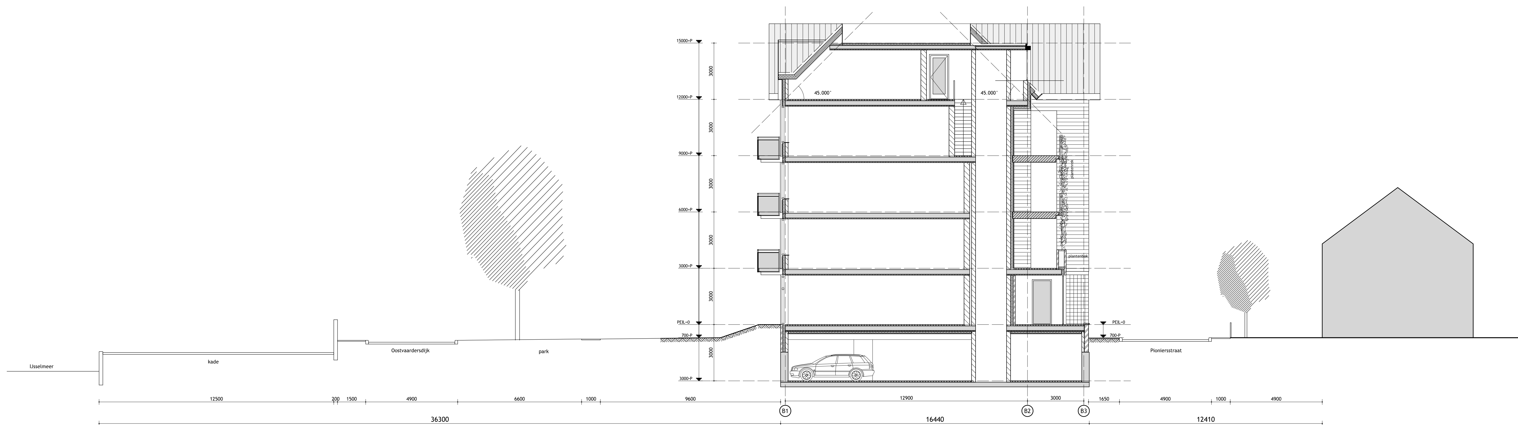
DOORSNEDE B-B
