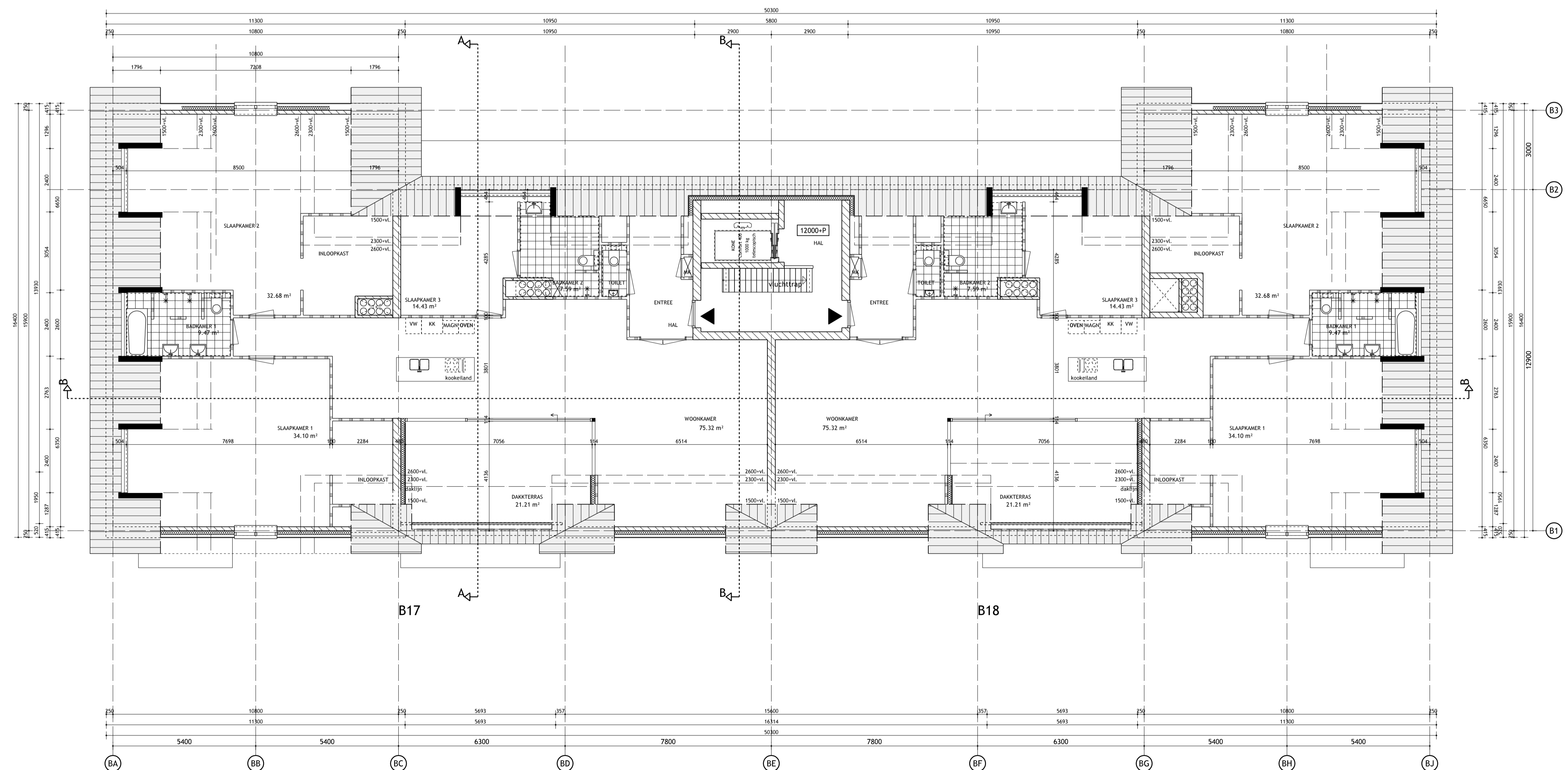
4e Verdieping gebouw B
